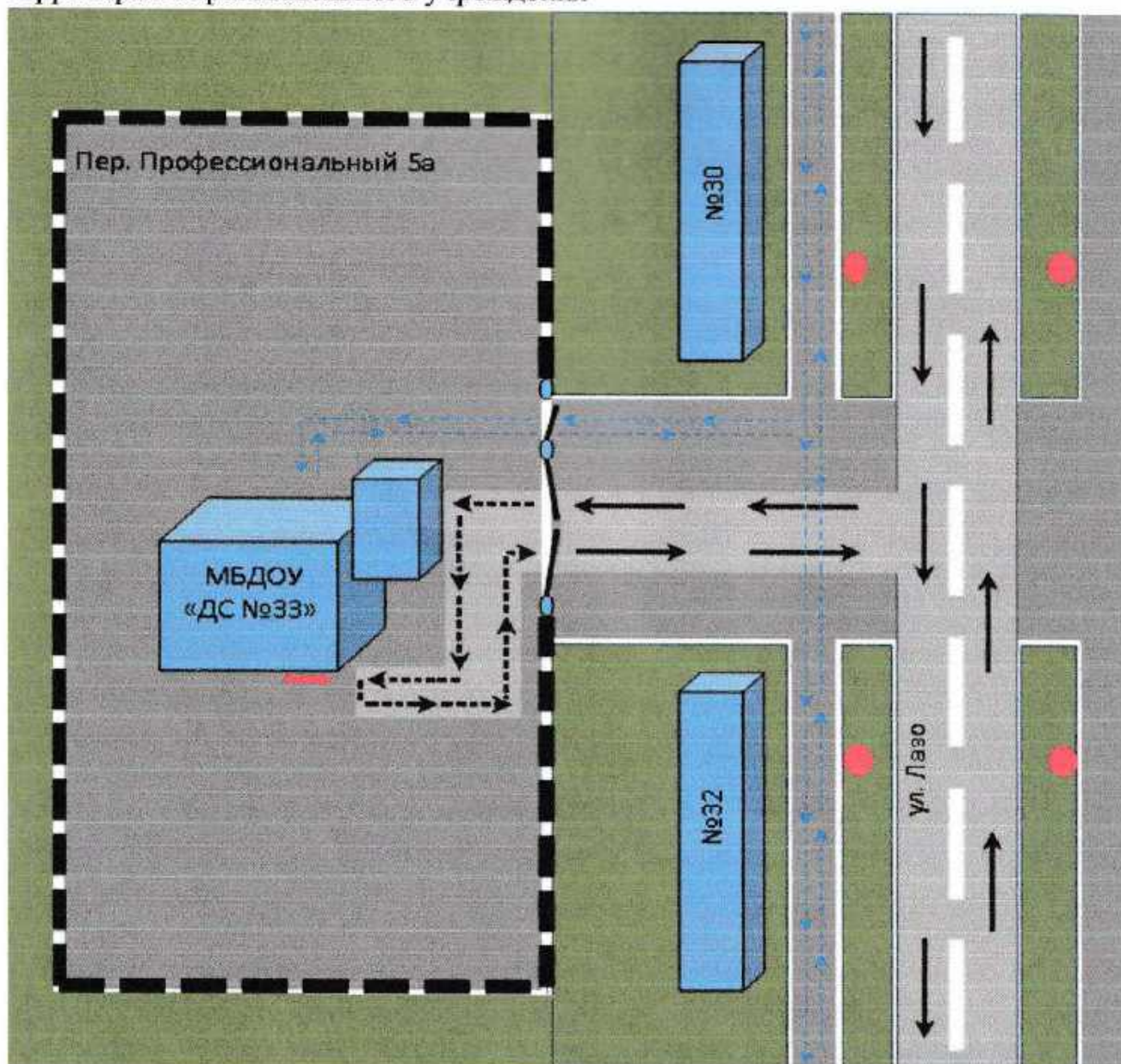
План-схема № 3 Пути движения транспортных средств к местам разгрузки/погрузки и рекомендованные пути передвижения детей по территории образовательного учреждения
